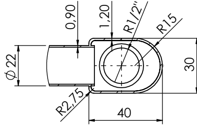
DETAY B ÖLÇEK 1 : 2
